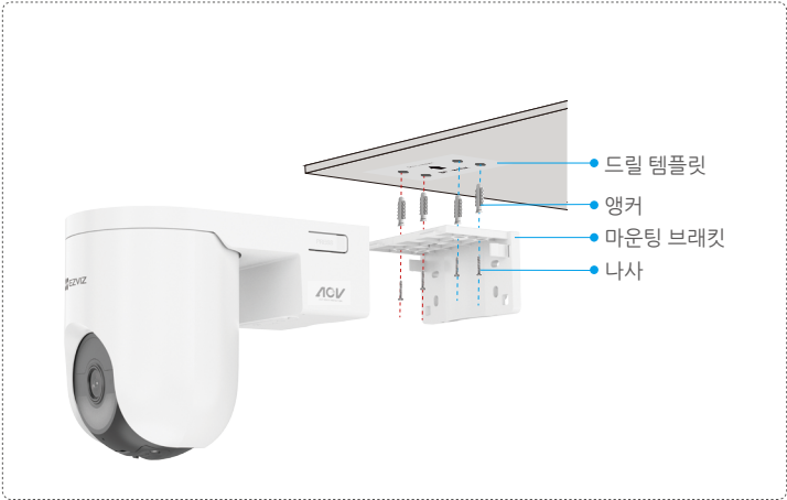
그림 1 천장 장착
